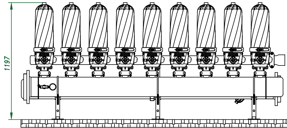
Вид спереди
