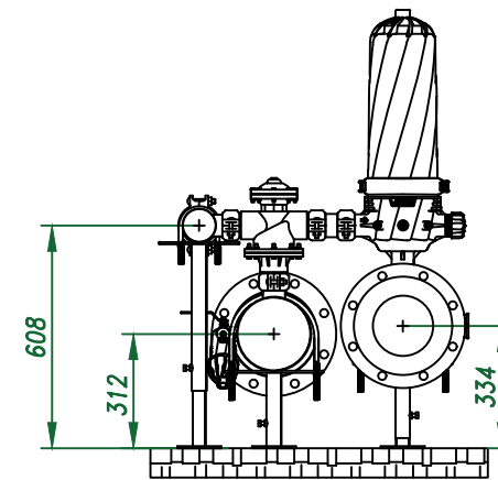
Вид слева
