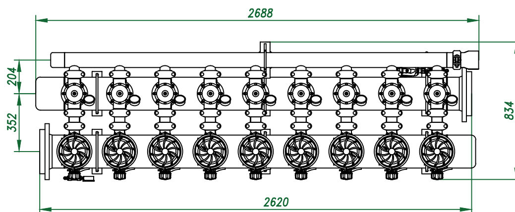
Вид сверху
